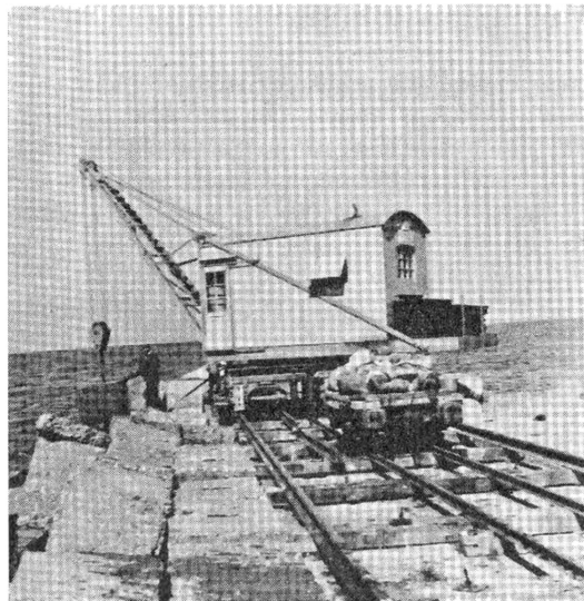
8-tonns kranen med kastninger i 1970.
