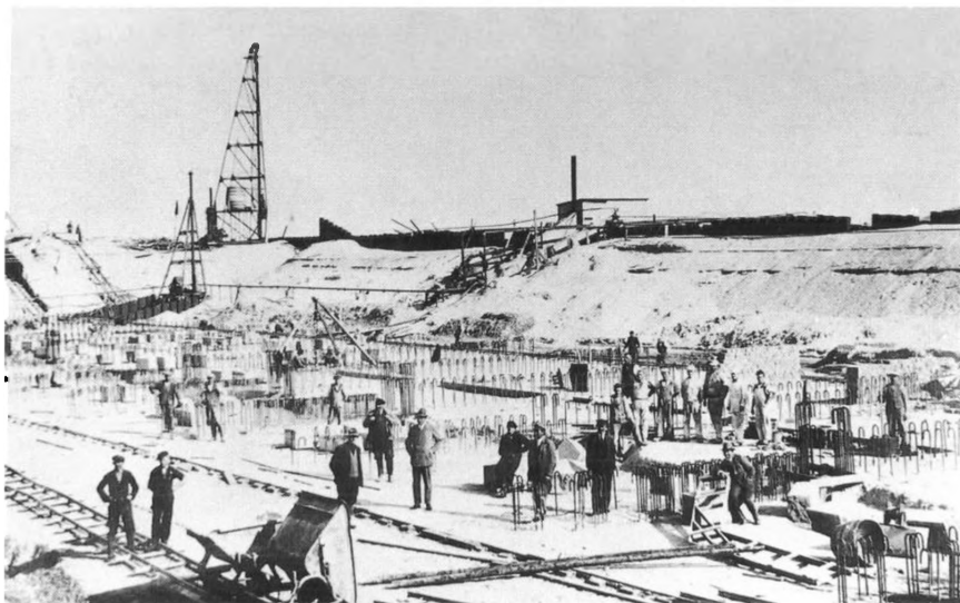
Den 1,70 meter tykke bund i afvandingslusen er færdigstøbt. I baggrunden sanddæmning og spunsjern, der værner byggegruben mod fjordvandet.
